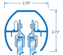
Precision Rollers
